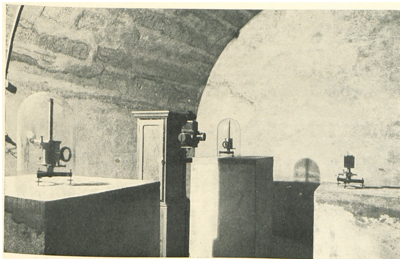
Enregistreurs magnétiques.
