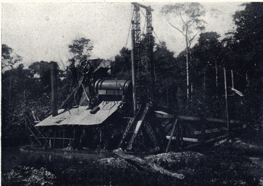
DRAGUE A OR TRAVAILLANT SUR UN PLACER SEC.
