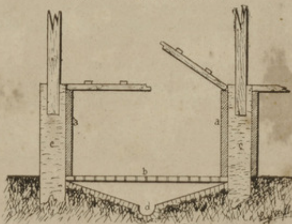
Fig. 2. — Élévation transversale.
