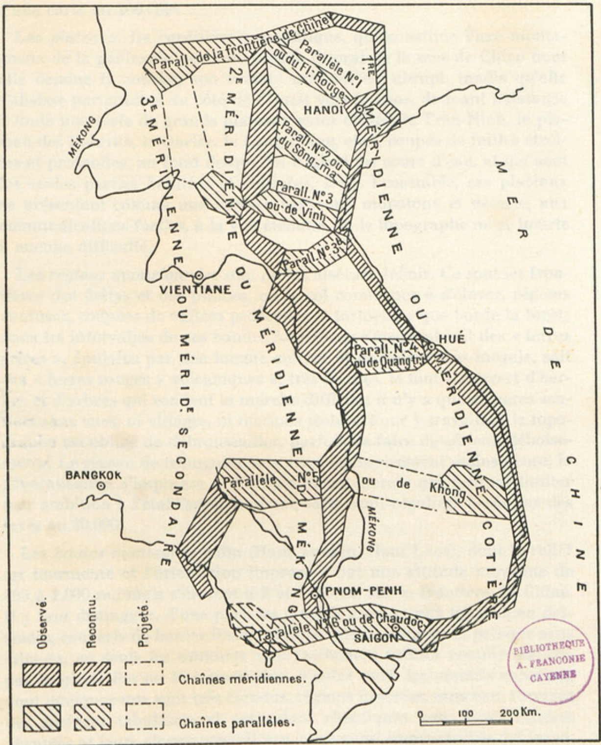
CANEVAS GÉODÉSIQUE D'ENSEMBLE DE L'INDOCHINE.
