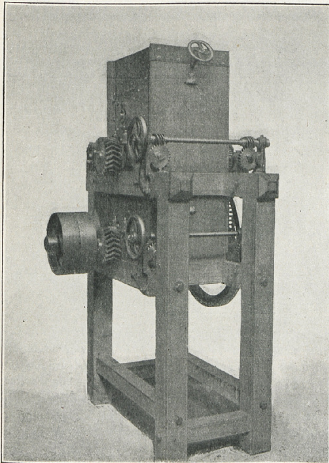
FIG. 46. — Broyeur de fécule verte.
