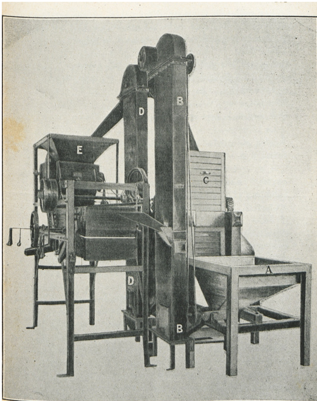
FIG. 50. — Appareil à tapioca comestible (système Hérault).
