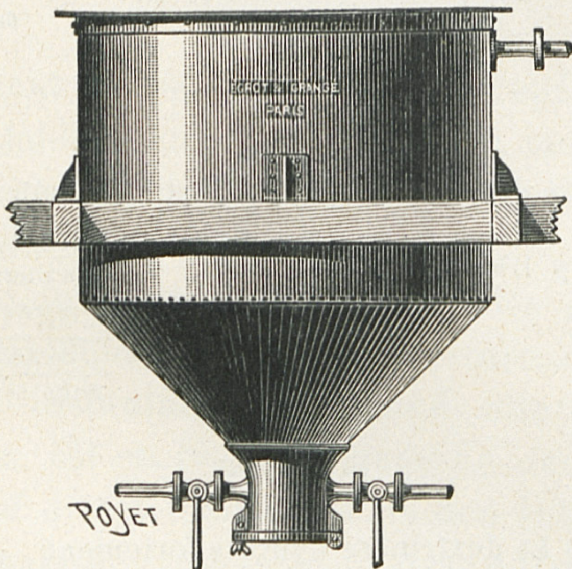
FIG. 58. — Cuve de trempage.
