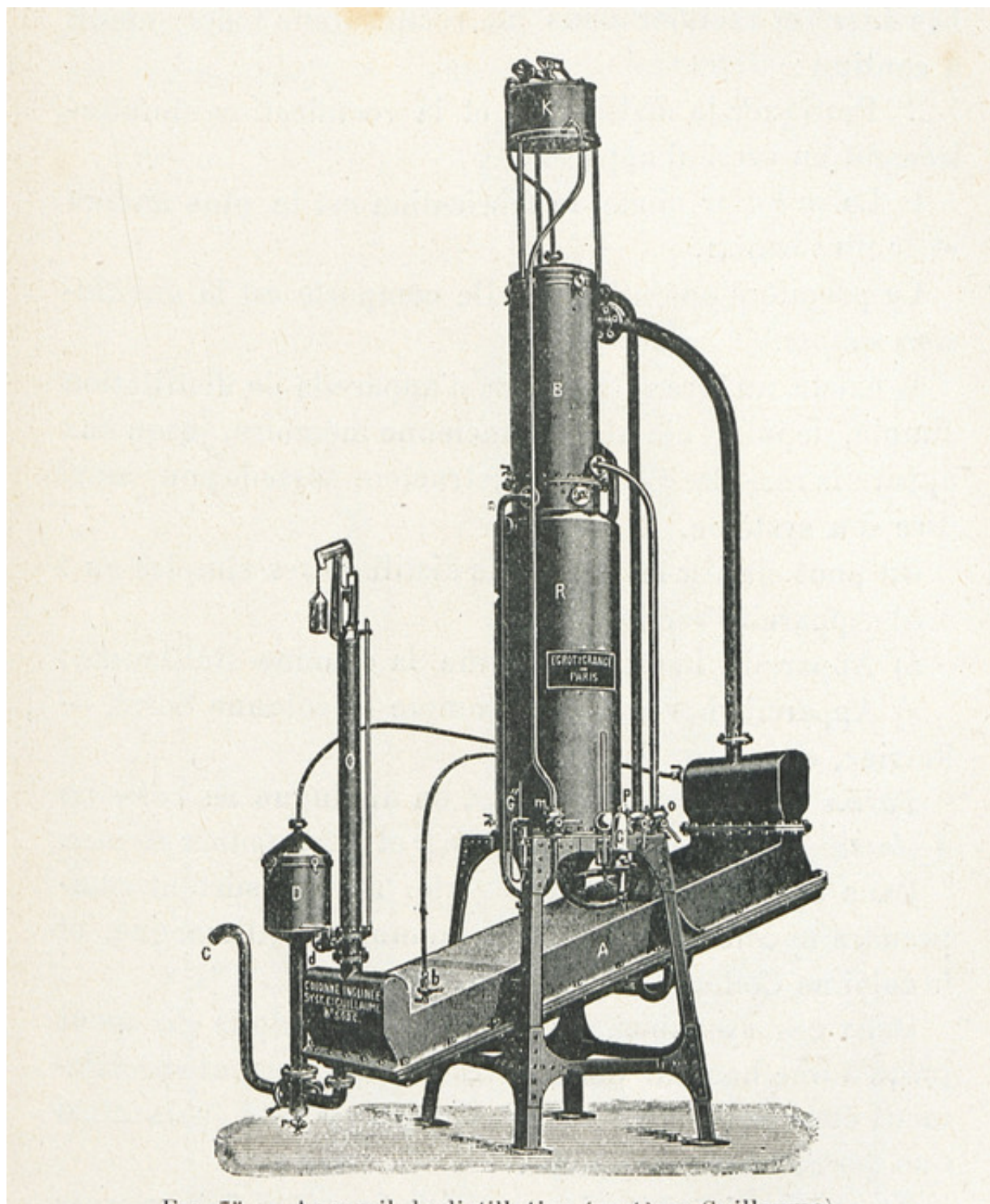
FIG. 75. — Appareil de distillation (système Guillaume).
