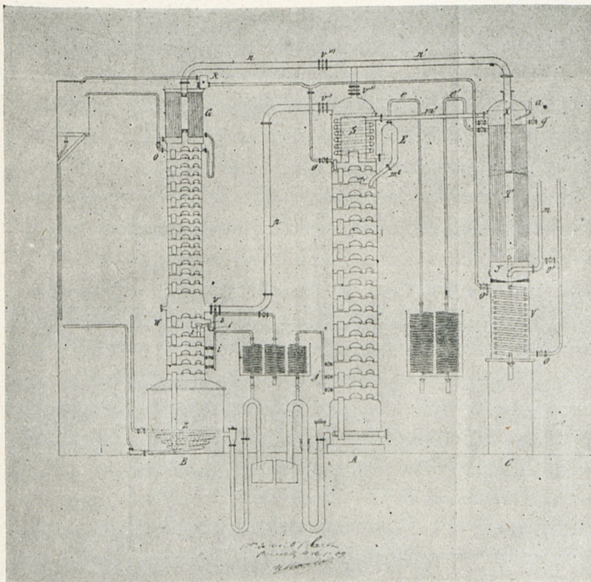
FIG. 87. — Appareil multidistillatoire (système O. Blaret).
