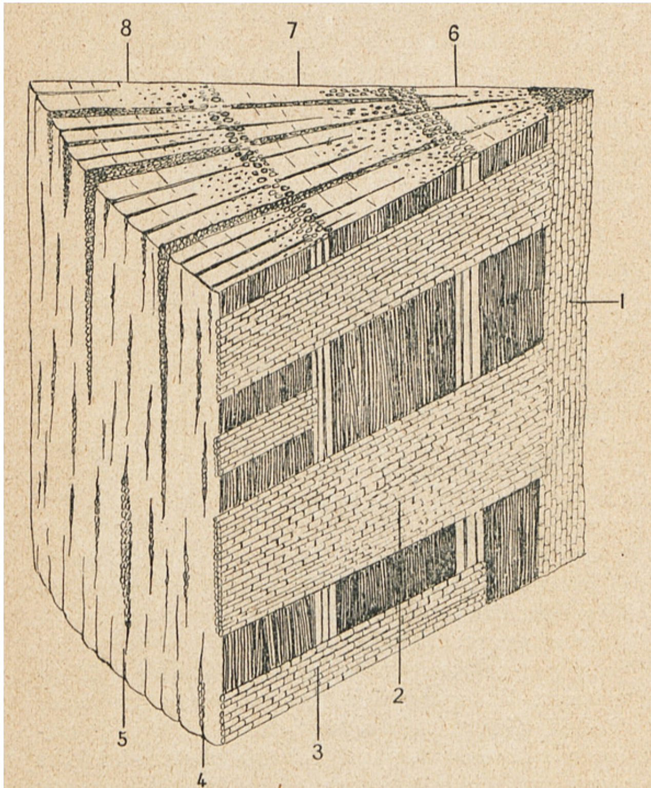
Fig. 6. — QUARTIER D'UNE TIGE DE CHÊNE DE TROIS ANS. — 1, moelle; 2, 3, rayons du bois; 4, 5, leur terminaison à la sur- face; 6, 7, 8, bois de première, deuxième et troisième année.
